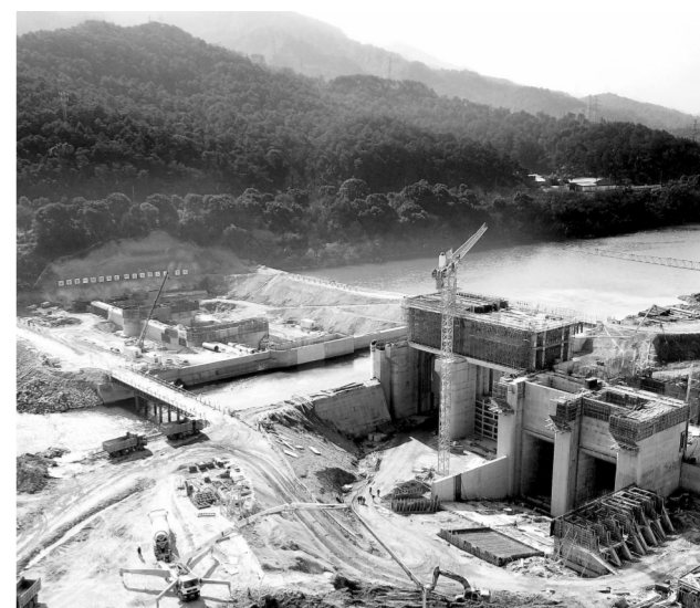
1月12日,正在紧张施工建设中的景德镇水利枢纽工程现场一片繁忙。该工程计划总投资4.51亿元,预计今年3月完成大坝主体工程建设。大坝坝线总长度310.10米,相应库容2840万立方米。
