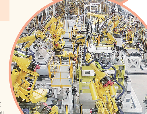
蜂巢能源锂电车间
