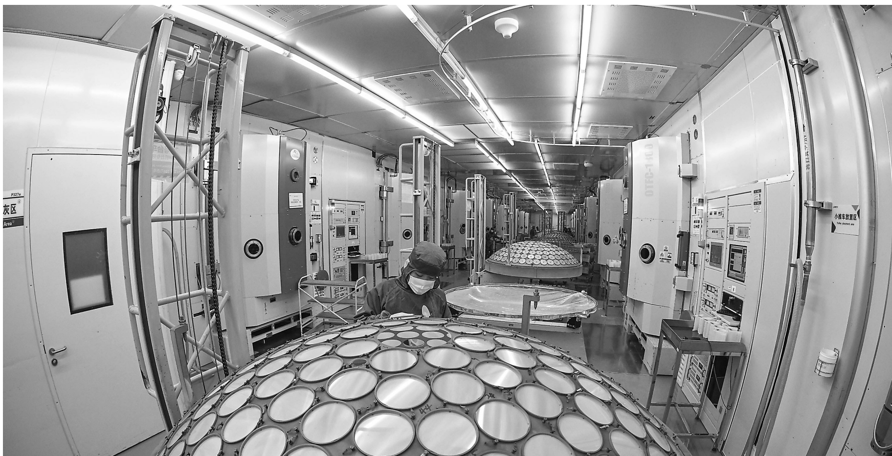
2月22日，位于南昌高新区的江西兆驰半导体有限公司蒸镀车间，员工正在蒸镀上片。
