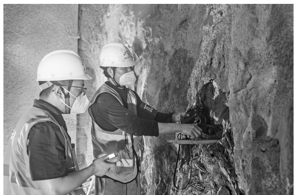
▲5月8日，中铁五局的建设者在渝昆高铁彝良隧道内进行瓦斯检测。
