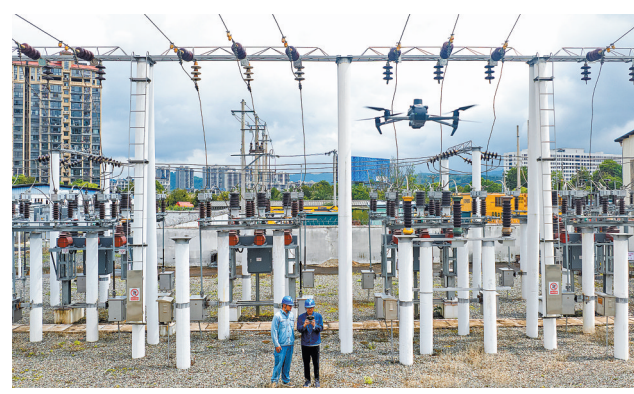
5月6日，国家电网安远县供电公司工作人员在修田村巡检变电设备，为居民筑牢入夏用电安全网。通讯员 刘思婷摄
