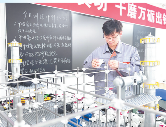
章琼正在进行甲烷氯化物单塔精馏装置的工艺流程设计与搭建。
