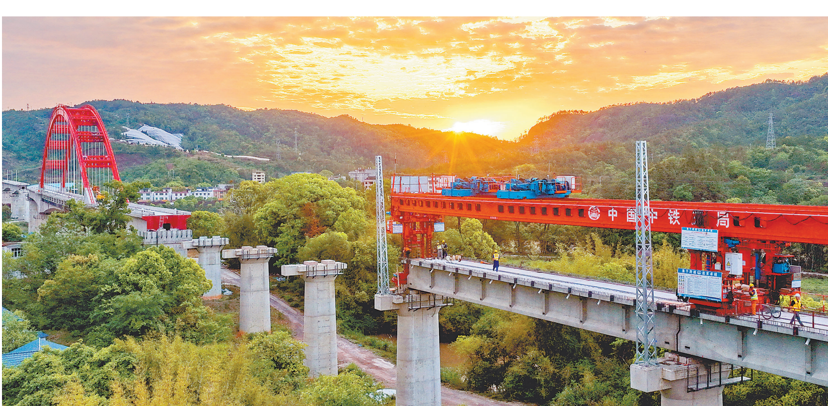
建设正酣 4月7日，会昌县文武坝镇林苏村，瑞梅铁路湘水特大桥连续梁架桥作业现场一片火热，建设者加紧施工，全力推进项目建设，为会昌段全线铺轨奠定基础。瑞梅铁路建成通车后，将结束我省寻乌、安远两县和广东省平远县无铁路历史。特约通讯员 朱海鹏摄
